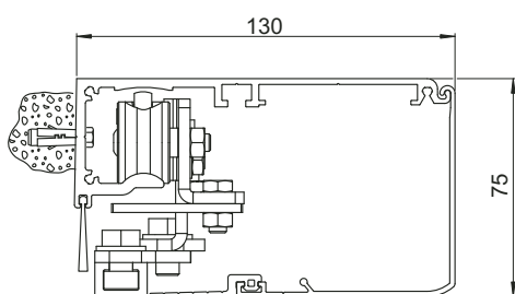
Civik - Querschnitt
